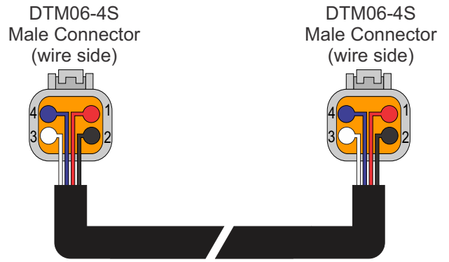
Haltech CAN cable wiring diagram
